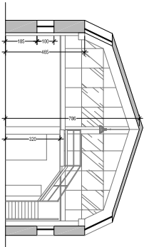
SEZIONE AA
